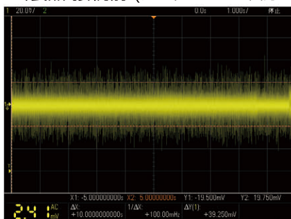
当製品 接続前 (ノートPCのUSB出力5V *USB-DC変換ケーブル経由にて)
