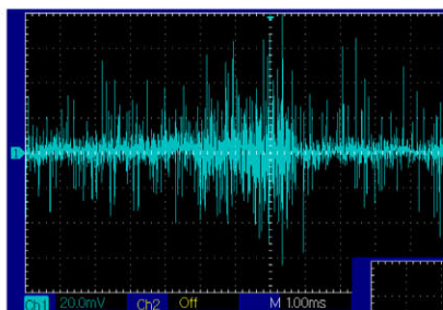
使用前 (可変スイッチング電源装置出力32V)
